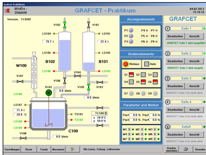
Simulierter Rührkesselreaktor
