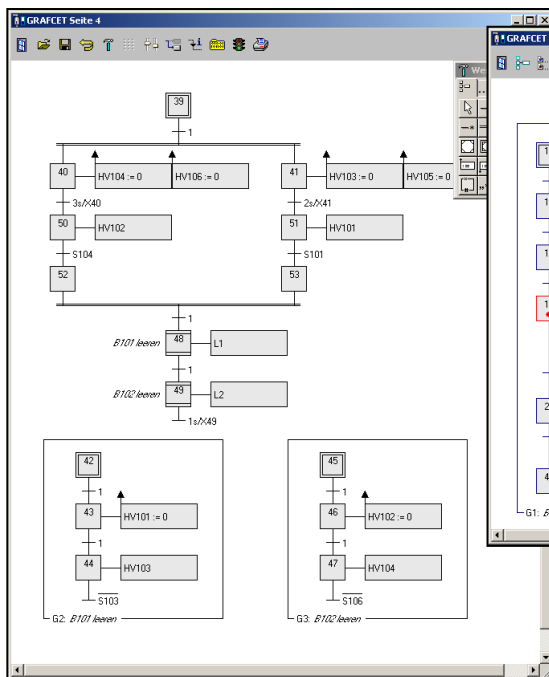
Editor zum Erstellen der GRAFCET-Pläne
