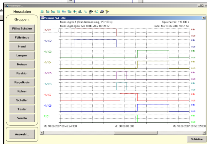
Trenddarstellung der Signalverläufe
