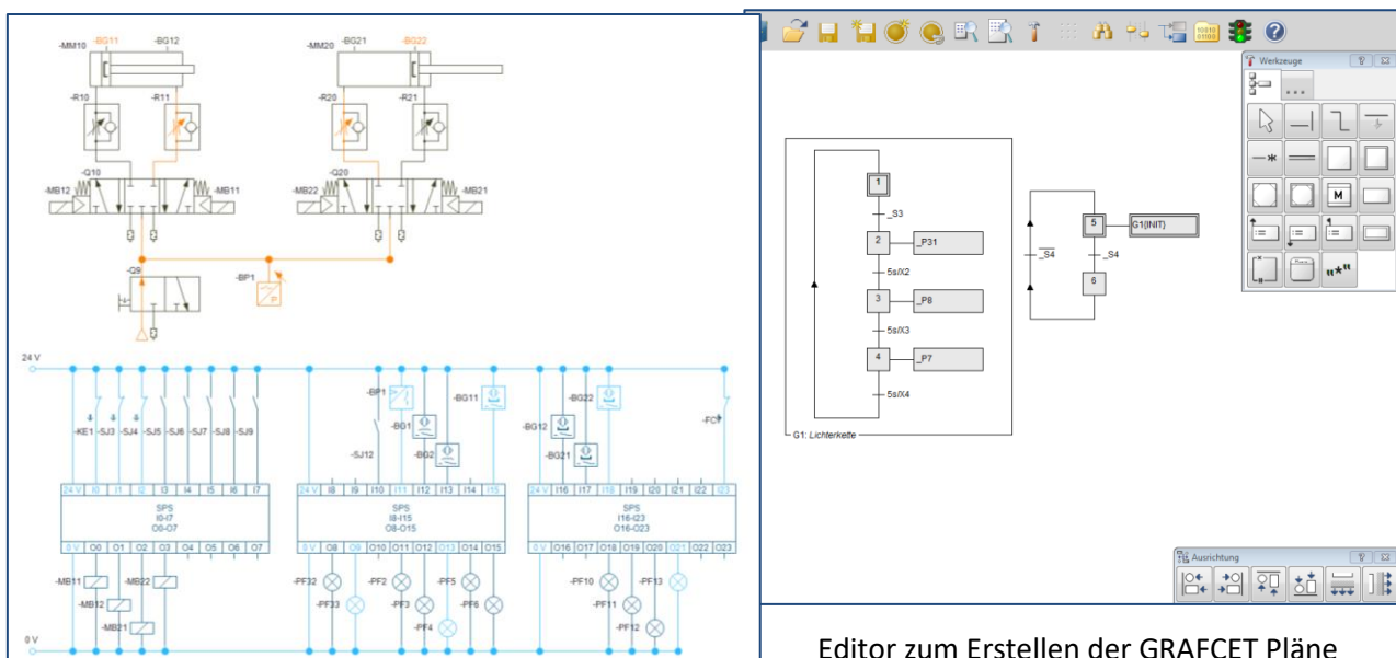
Elektropneumatische Überwachung der Ventile
