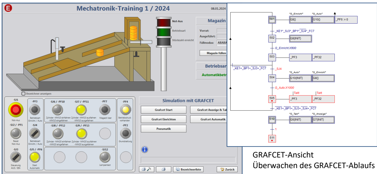
Simulierte Mechatronik-Anlage
